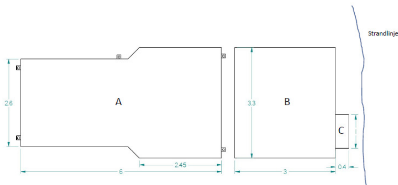
Bild 1 visar måttsett planritning av aktuell brygga efter ombyggnad och borttagande ca 8 meter av bryggans nuvarande längd om 17,7 meter till 9,7 meter.
