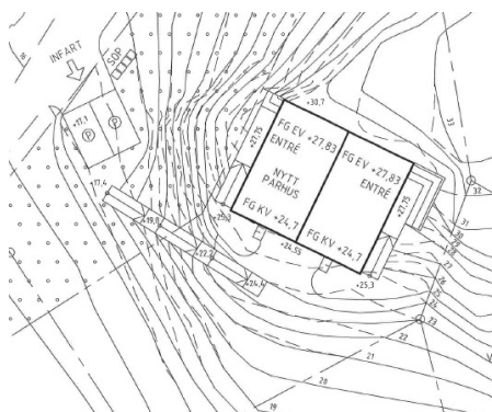
Bild 1 Utdrag från bygglövsritning
