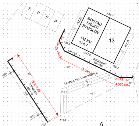
Bild 2 redovisning av tillkommande murar 19,28+26,13 = 45,41 löpmeter
