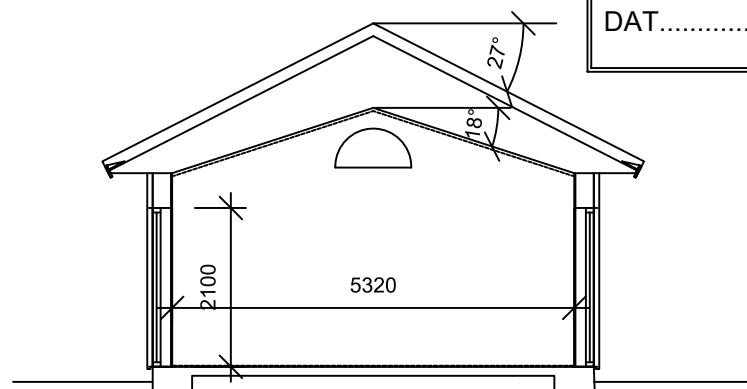
SEKTION B-B
