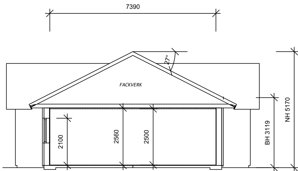
SEKTION A-A
