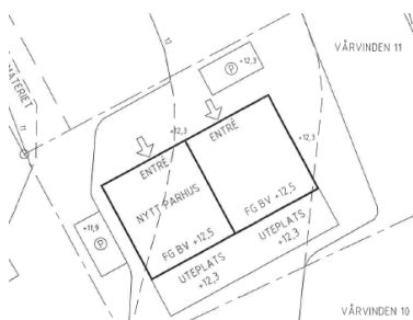
Bild 1 Utdrag från bygglövsritning
