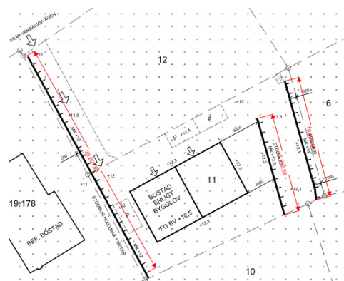
Bild 2 redovisning av tillkommande mur 1 19,4 meter mur 2 15,8 meter och mur 3 39 meter totalt = 74,2 löpmeter
