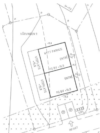
Bild 1 Utdrag från bygglovsritning
